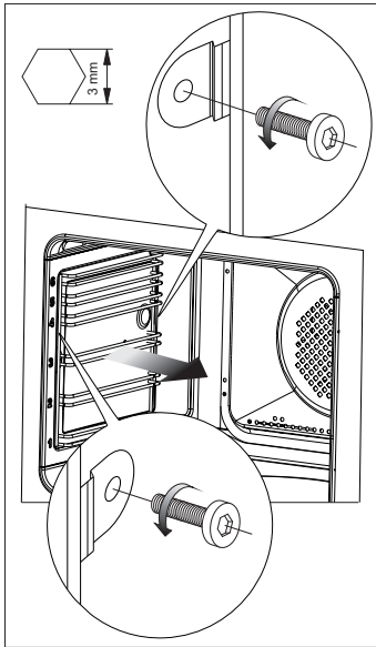
Vyjímání drátěných vodicích lišt
