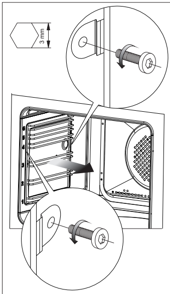
Vyberanie drôtených vodiacich lišt
